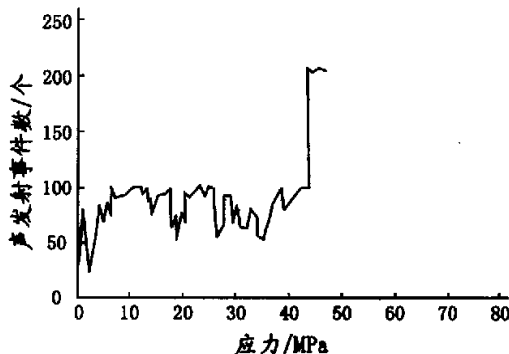
图 2 声发射事件数—应力曲线
